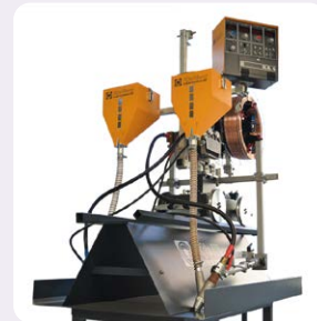
Modifikation für das Schweißen von Trapezblechen
