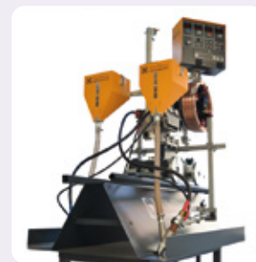
Modifikation für das Schweißen von Trapezblechen
