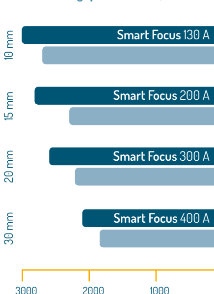
Schneidgeschwindigkeit mm/min, Baustahl Cutting speed mm/min, mild steel
