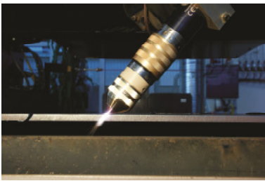
Bild 4: Fasenschneiden in höchster Qualität mit Plasmaschneidtechnik von Kjellberg Finsterwalde
