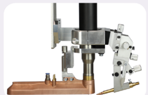
Schleppgasdüse mit Brenner
