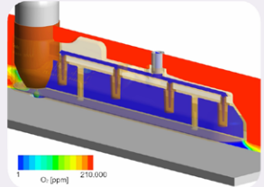
Sauerstoffmessung
